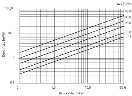
Kapazitätsdiagramm - 0,7 mm
