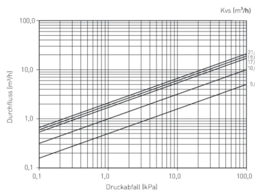
Kapazitätsdiagramm - 0,5 mm
